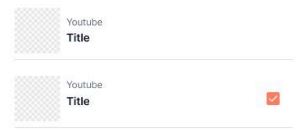
Thumbnail Item
