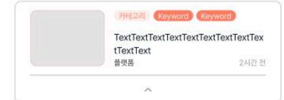
Thumbnail Item_main
